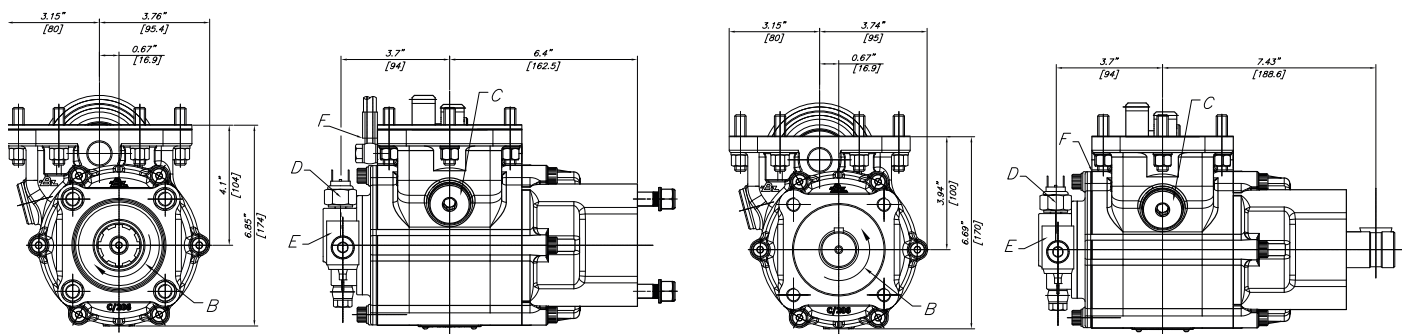
Round shaft Eje chaveteado
