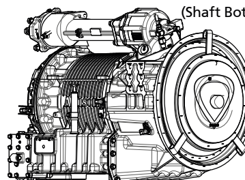
4000 (EVS /MH /RDS /TRV) 4500 (EVS /RDS) + Retarder P/N. 9076599
